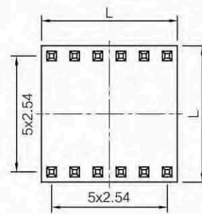
12 контактов
