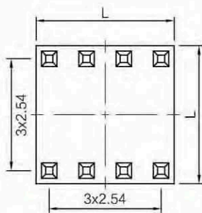
8 контактов
