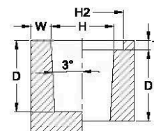
Сквозное или глухое отверстие, конусность=3°
